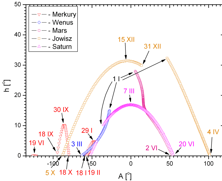
Jasne planety na początku świtu cywilnego (Słońce 6° pod horyzontem)
