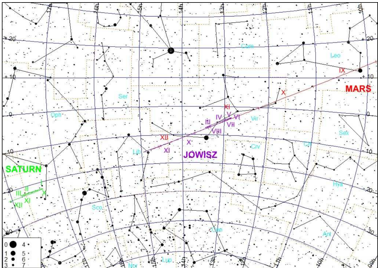
Trasy Marsa, Jowisza i Saturna na tle gwiazd w 2017 roku.
