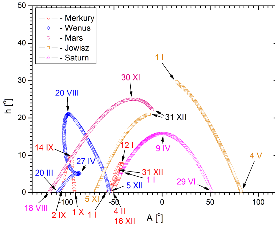
Jasne planety na początku świtu cywilnego (Słońce 6^\circ pod horyzontem)
