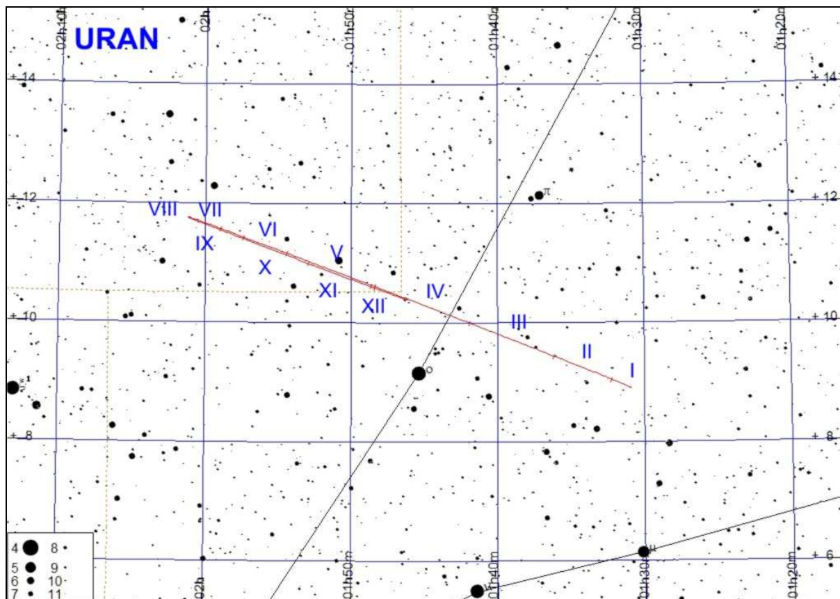
Trasa Urana na tle gwiazd w 2018 roku.
