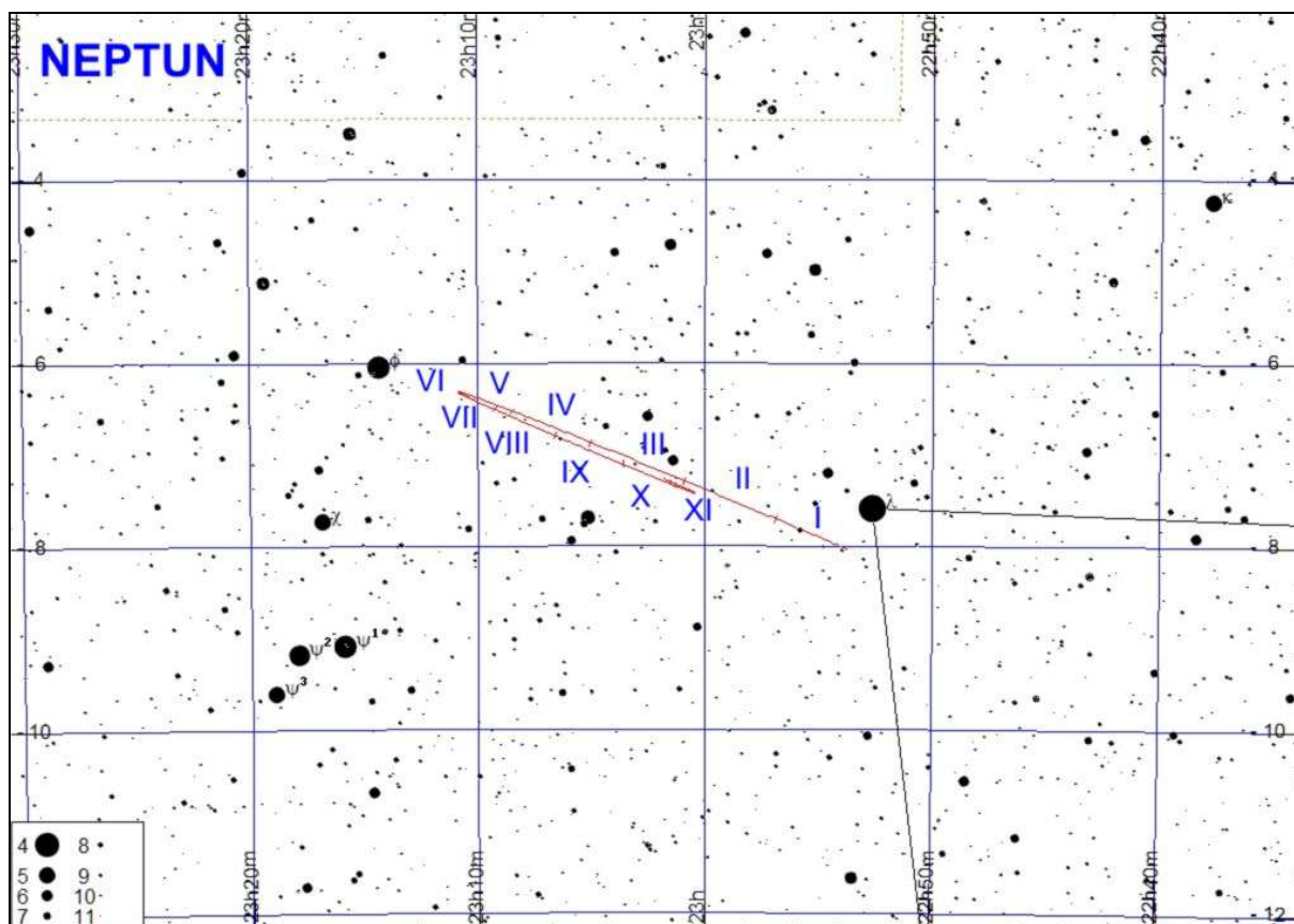
Trasa Neptuna na tle gwiazd w 2018 roku.
