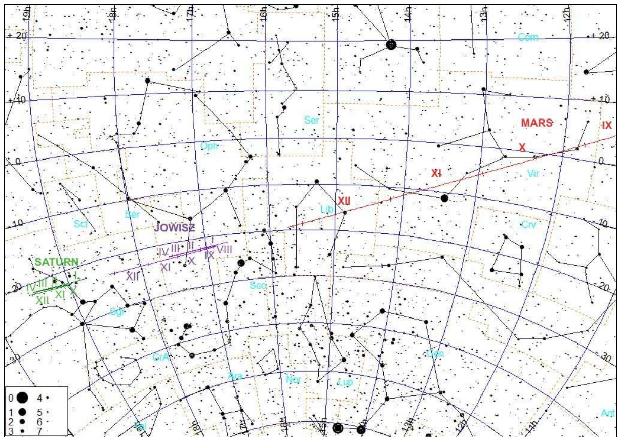
Trasa Marsa, Jowisza i Saturna na tle gwiazd w 2019 roku.
