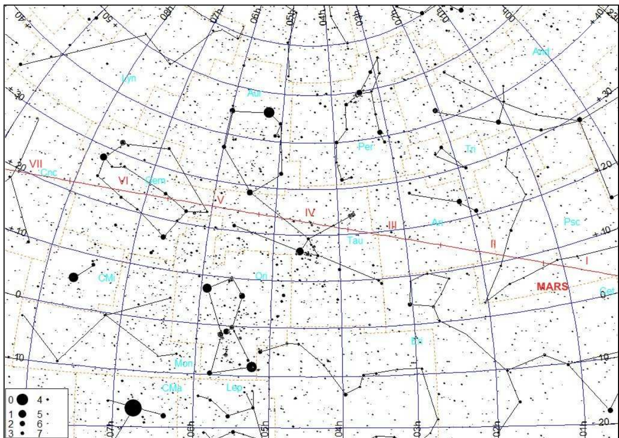
Trasa Marsa na tle gwiazd w 2019 roku.
