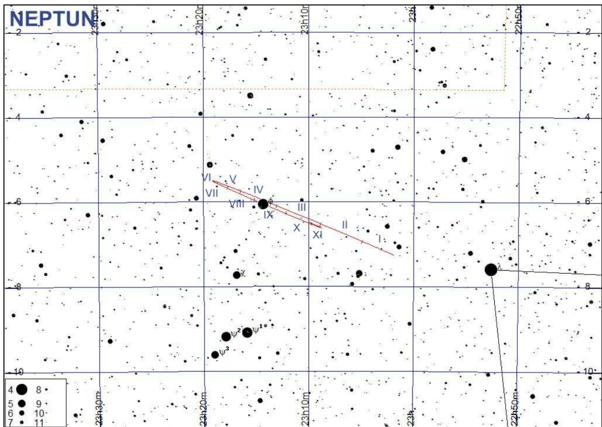
Trasa Neptuna na tle gwiazd w 2019 roku.
