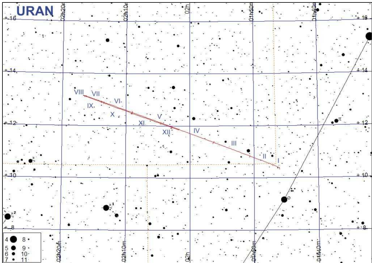
Trasa Urana na tle gwiazd w 2019 roku.
