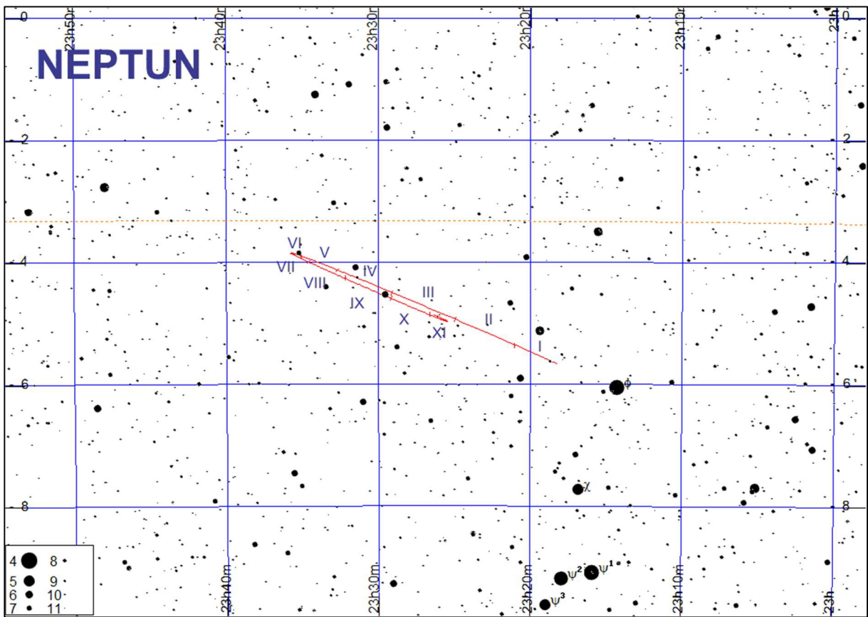
Trasa Neptuna na tle gwiazd w 2021 roku.
