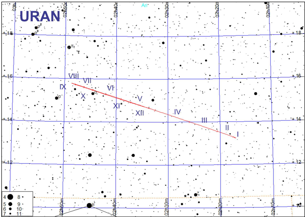
Trasa Urana na tle gwiazd w 2021 roku.
