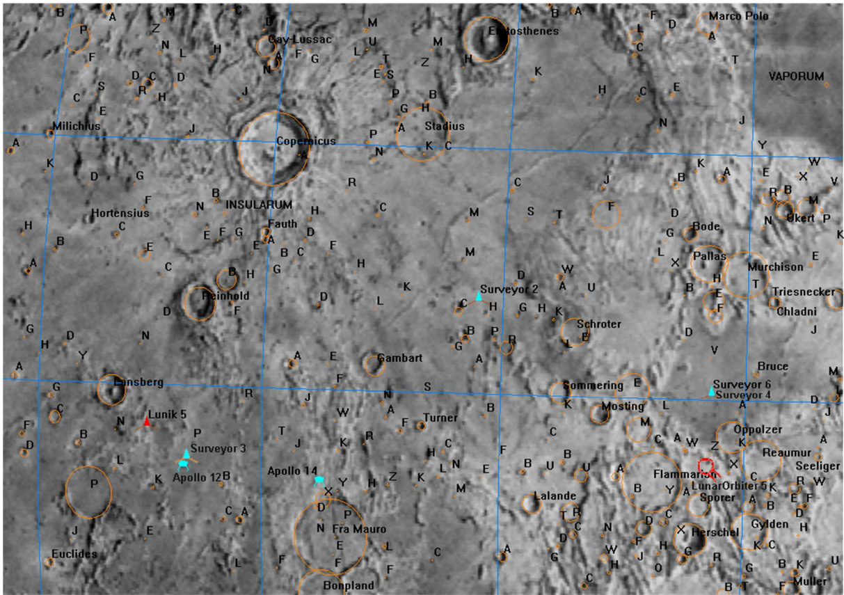
9. Kopernik (Copernicus)
