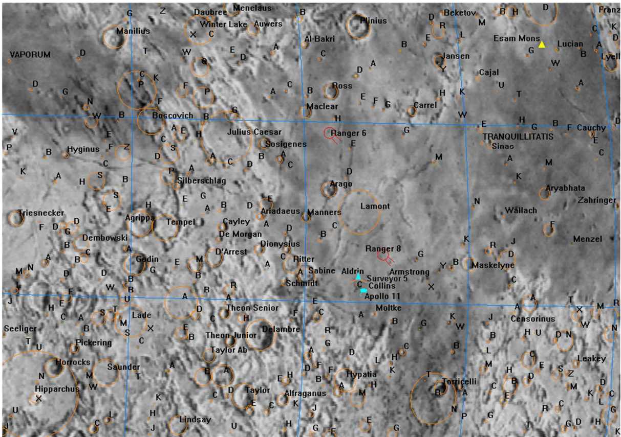
10. Morze Spokoju (Mare Tranquillitatis)
