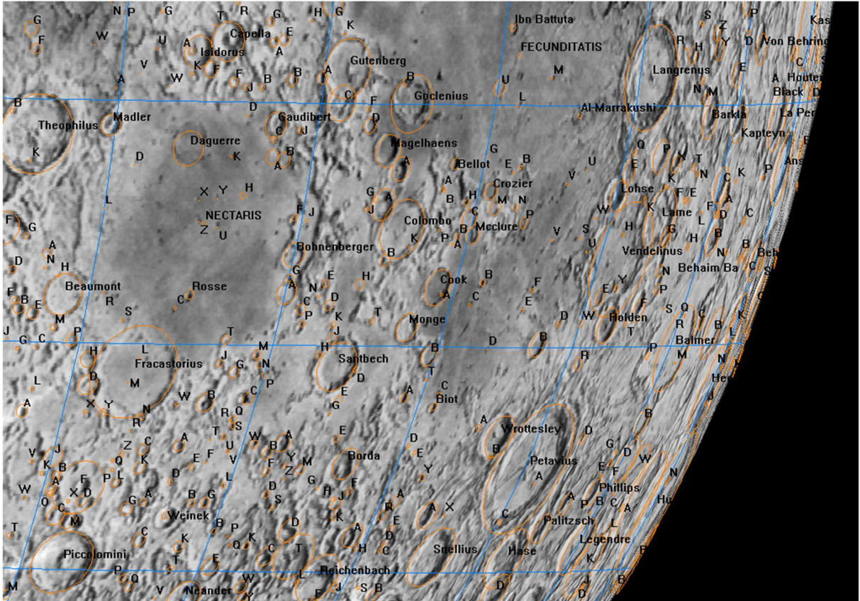
15. Morze Nektaru (Mare Nectaris)
