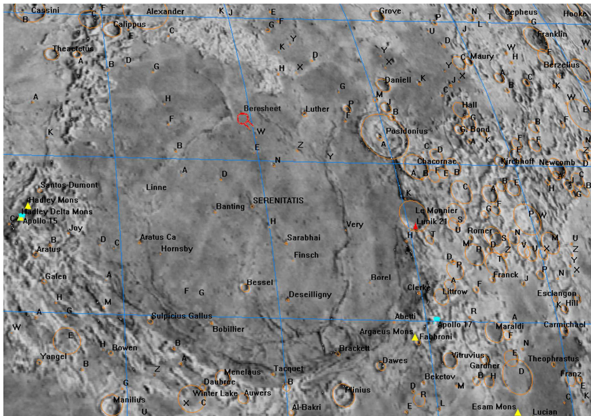
6. Morze Jasności (Mare Serenitatis)
