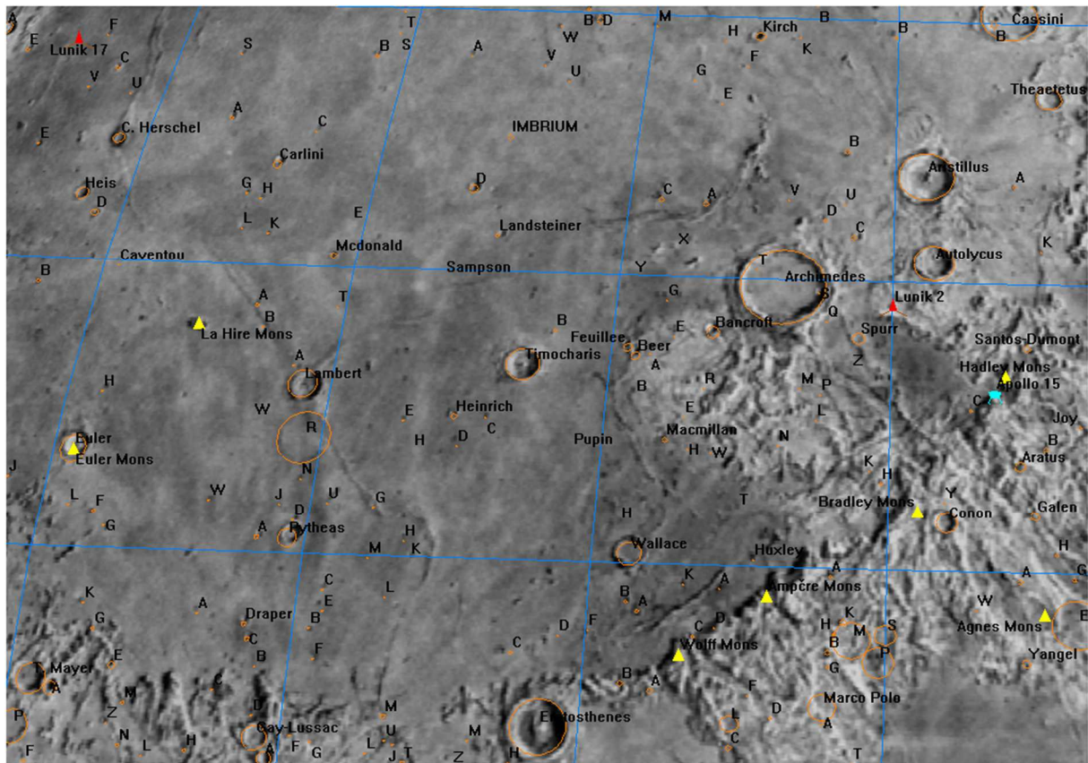
5. Apeniny
