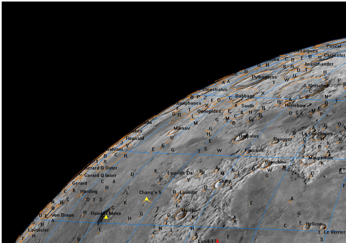
1. Zatoka Tęcz (Sinus Iridium)
