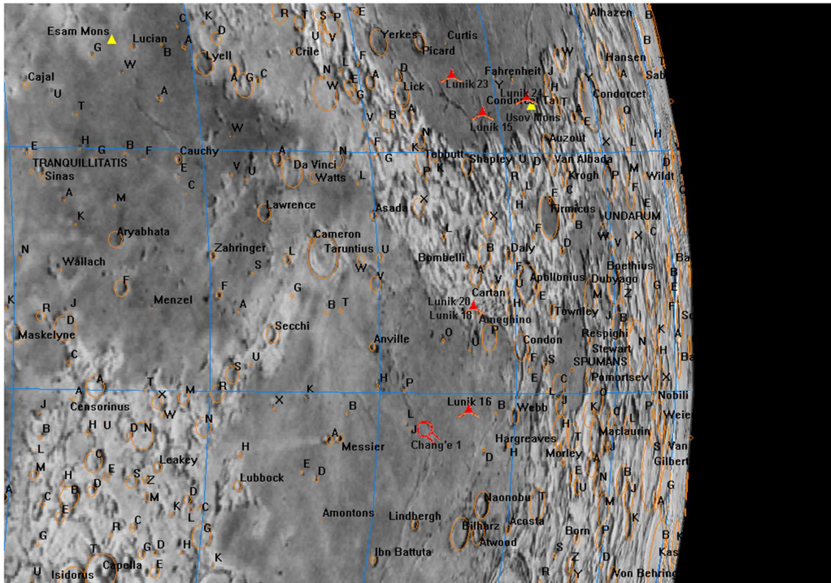
11. Morze Żyzności (Mare Fecunditatis)
