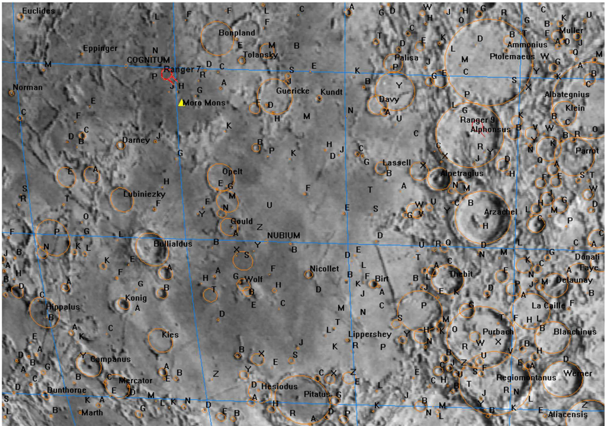
13. Morze Chmur (Mare Nubium)
