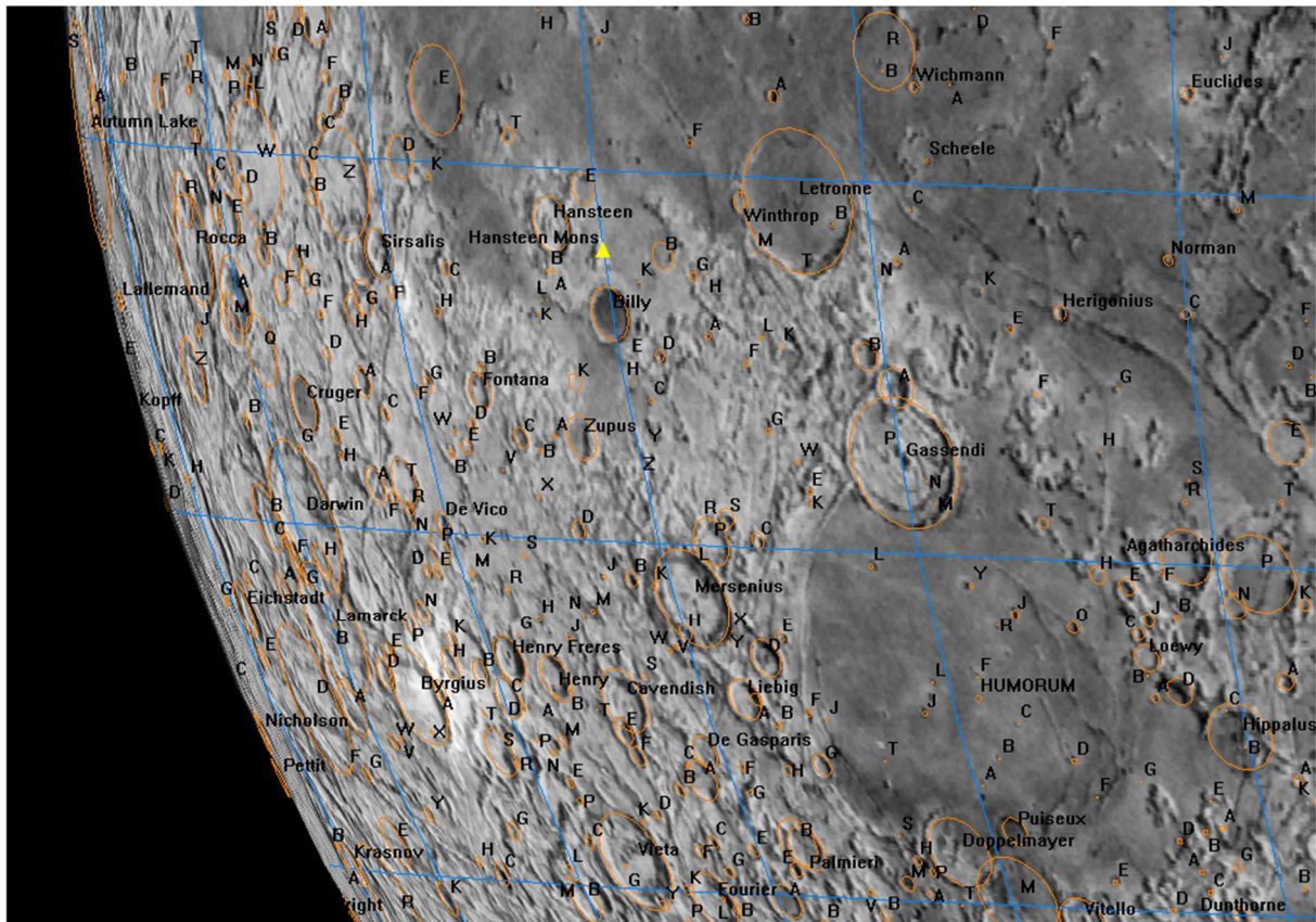
12. Morze Wilgoci (Mare Humorum)
