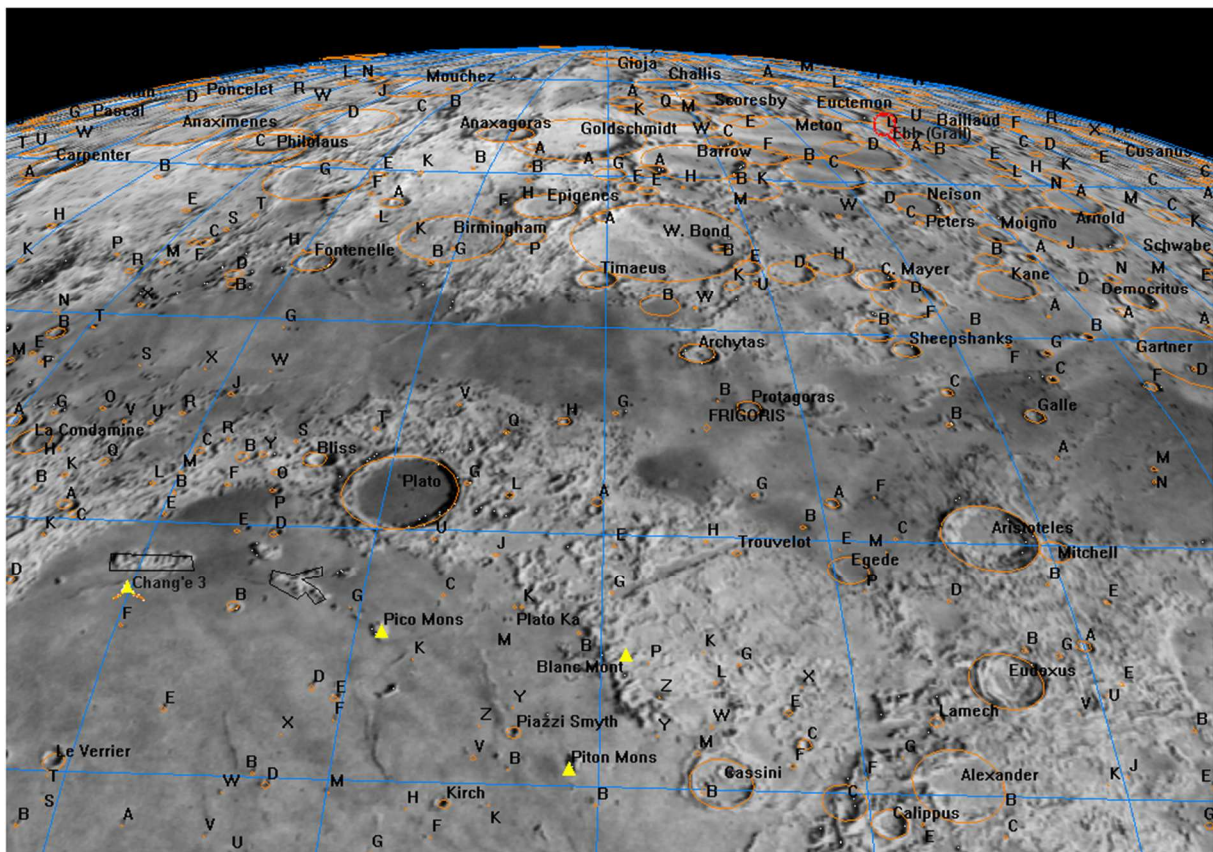
2. Alpy
