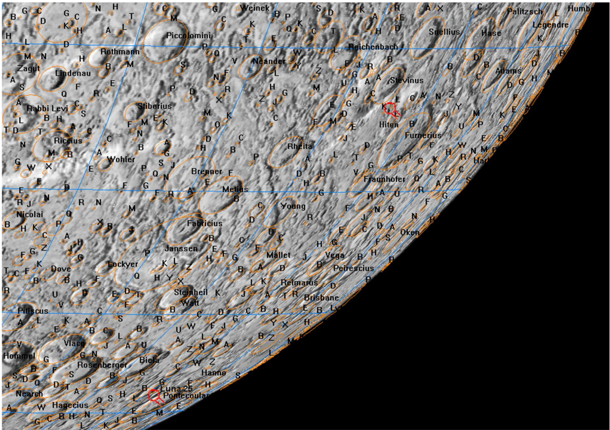
19. Fraunhofer
