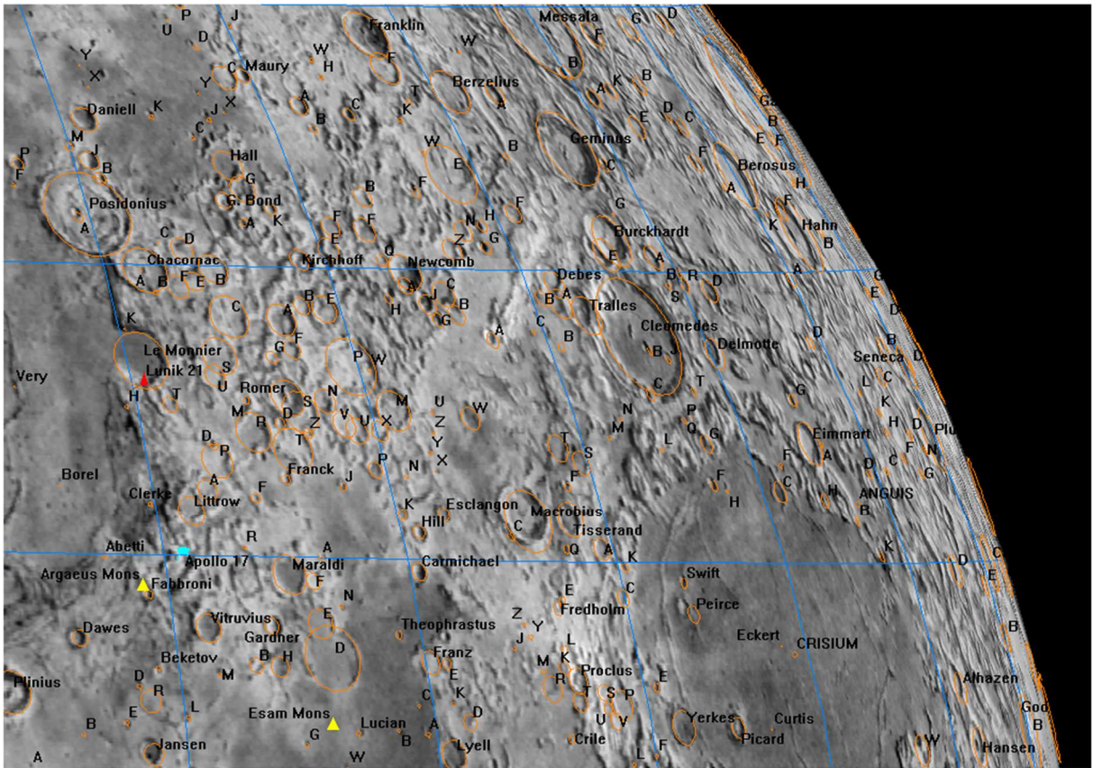
7. Morze Przesień (Mare Crisium)
