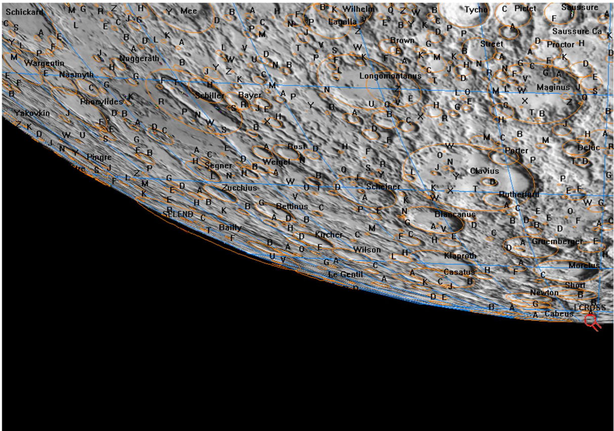
20. Clavius
