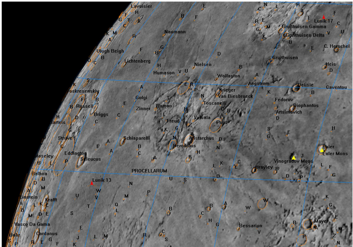
4. Ocean Burz (Oceanus Procellarum)
