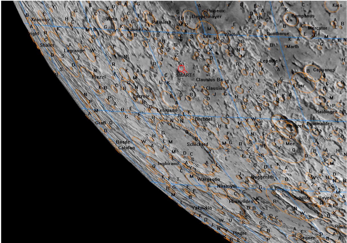
16. Schickard
