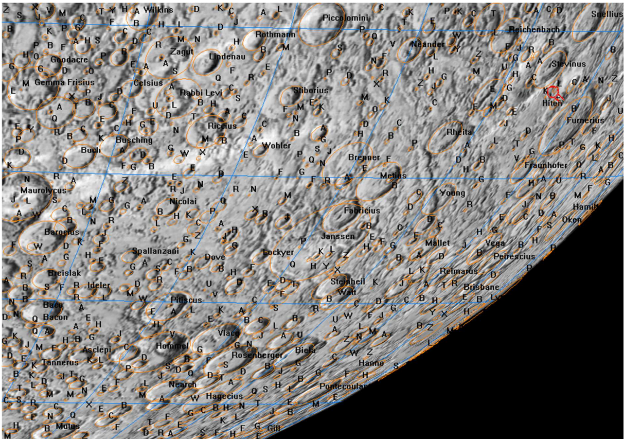
18. Piccolomini
