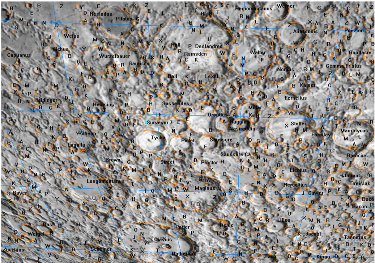
17. Tycho
