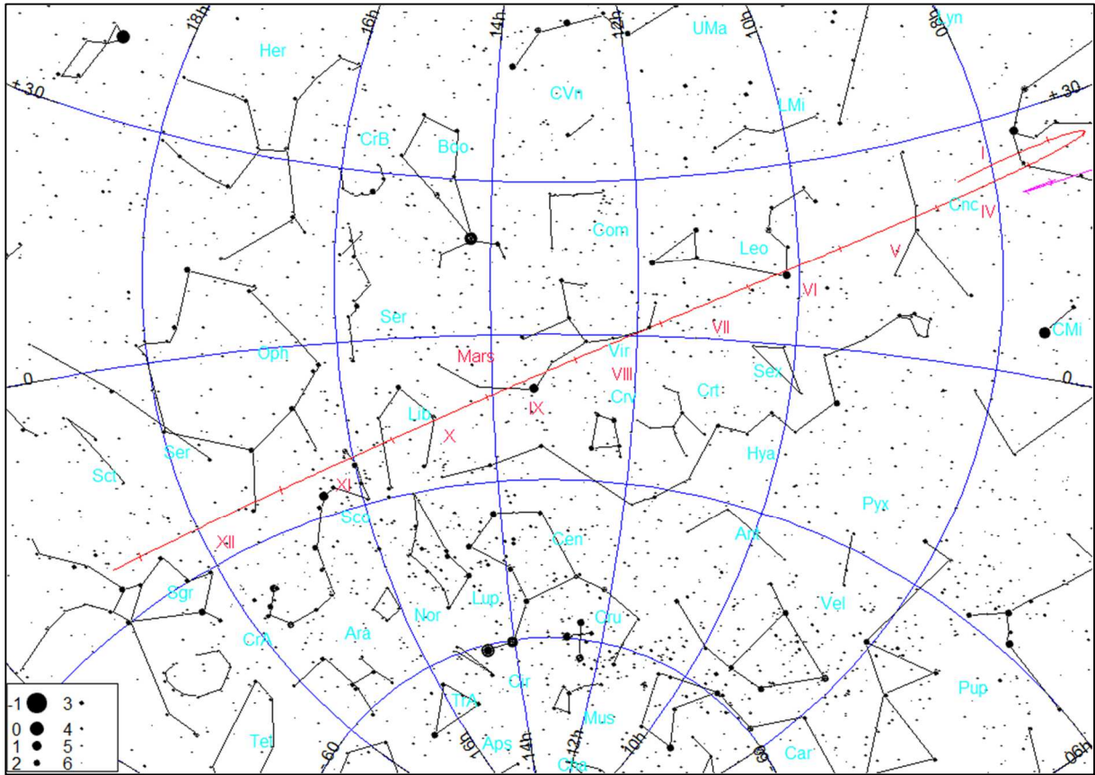
Trasa Marsa na tle gwiazd w 2025 roku.
