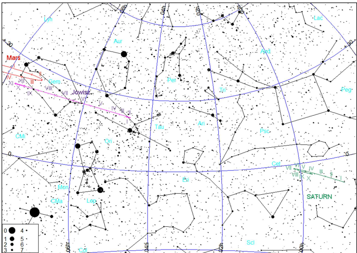
Trasa Jowisza, Saturna i Marsa na tle gwiazd w 2025 roku.
